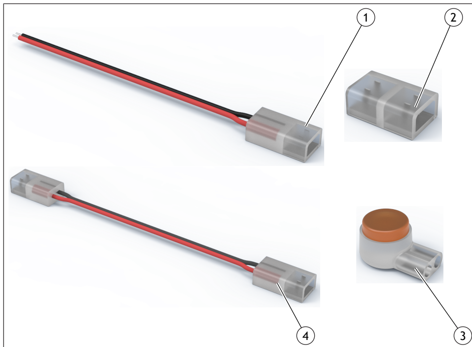
Abb. 3: LED-Band IP00 Zubehör
